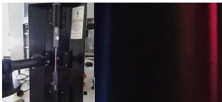
Εικόνα 1 Φως εκπνεόμενο από μια λάμπα που περιέχει αέριο Υδρογόνο και το αντίστοιχο φάσμα του.
